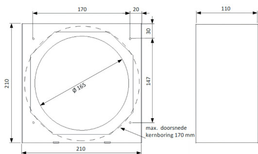
Compensatiekader in voor- en zijaanzicht
