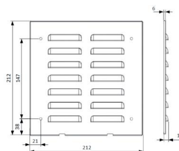
Beschermrooster Light in voor- en zijaanzicht
