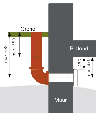
Voorbeeld inbouwsituatie MoveAir CELLAR
