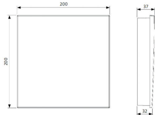
Afdekkap binnen bovenkant in voor- en zijaanzicht
