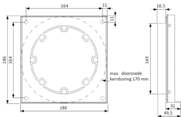
Afdekkap binnen onderkant in voor- en zijaanzicht
