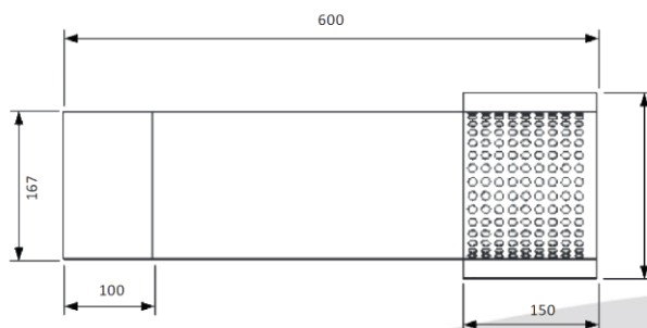
Afdekkap buiten (90° gedraaid) in vooraanzicht
